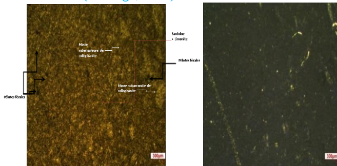
Figure 6. Phosphate de Kanzi au microscope (à gauche avec la lumière naturelle et à droite avec la lumière polarisée)
