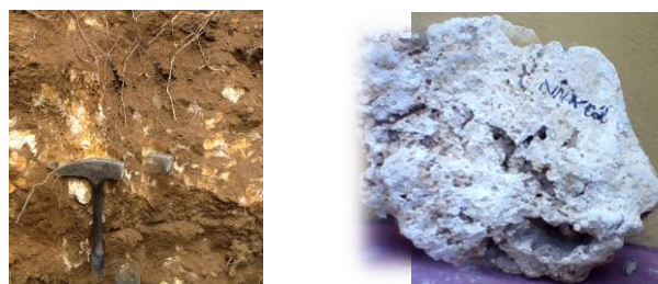
Figure 4. Phosphate de Kanzi vu sur terrain
