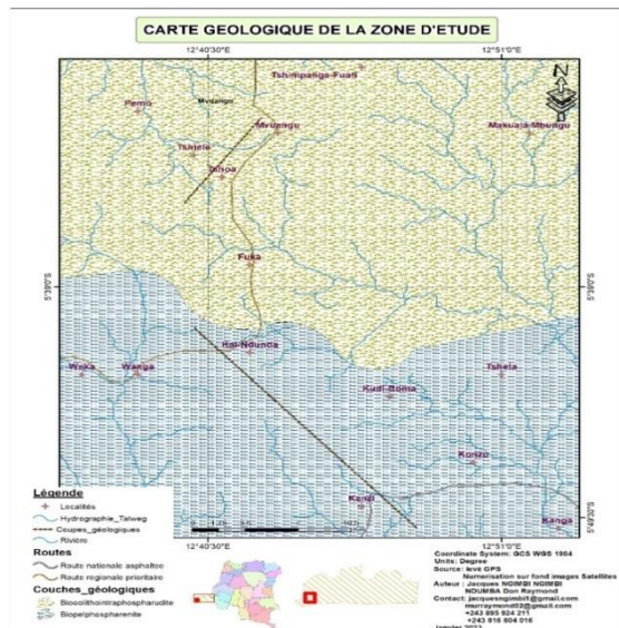
Figure 2. Carte géologique la zone d'étude
